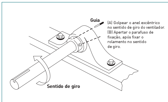
Figura 3. Conjunto do mancal de rolamentos
