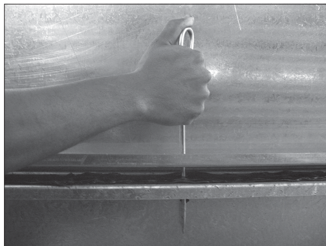
Figura 10. Introdução dos pinos-guia (alavanca tipo espina)
